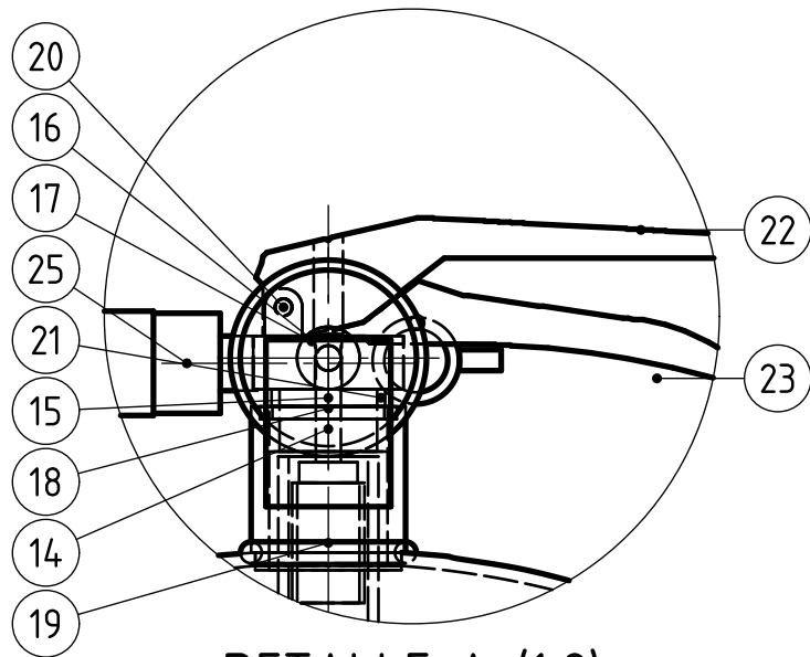
DETALLE A (1:2) Válvula, manómetro y manijas
