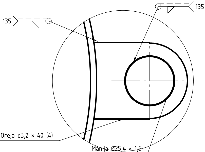
DETALLE G (1:1) Oreja de la manija (vista superior)
