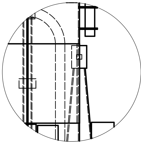
DETALLE E (1:5) Válvula esférica y tobera
