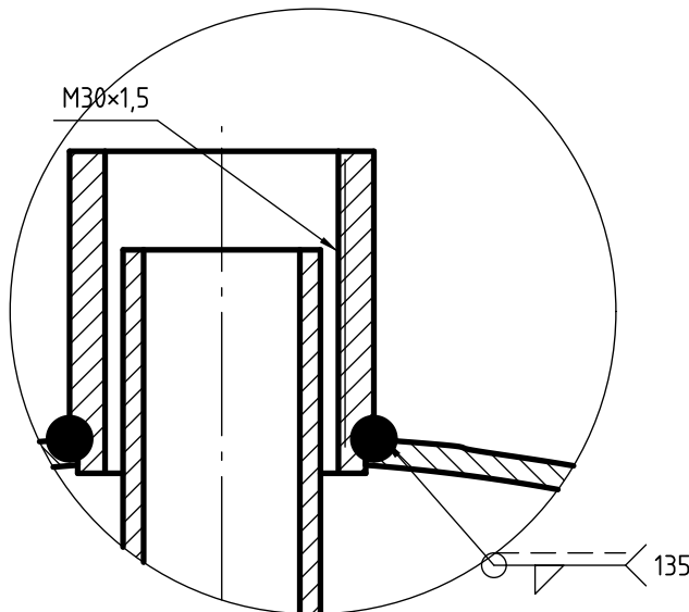
DETALLE B (1:1) Cupla soldada
