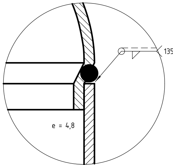
DETALLE C (1:1) Casquete con borde reducido y tope
