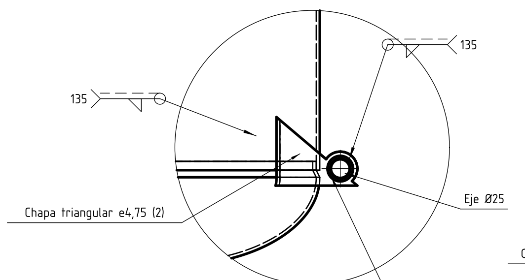
DETALLE F (1:5) Portaeje y chapa triangular (vista lateral, sin rueda)
