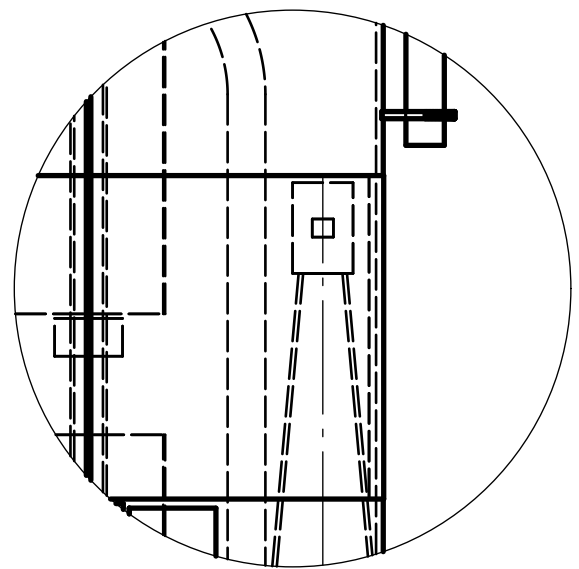
DETALLE E (1:5) Válvula esférica y tobera
