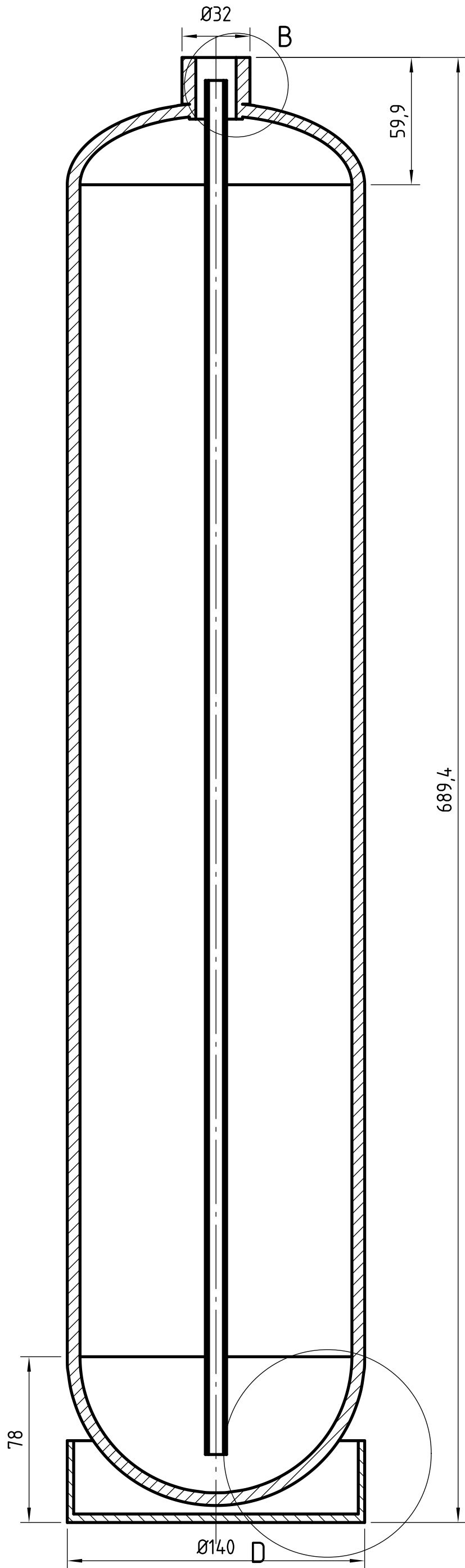
CORTE A-A (1:2)
