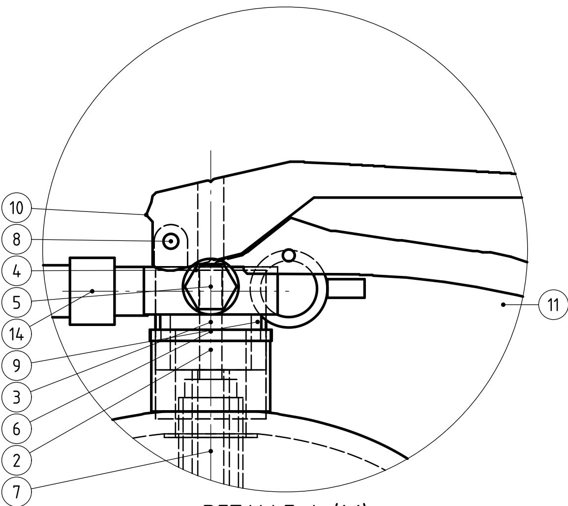
DETALLE A (1:1) Válvula, disco de seguridad y manijas
