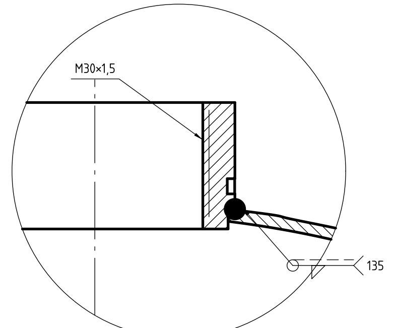
DETALLE B (2:1) Cuello roscado muesca de altura 2 × 1 × 2 (prensa Pannier); filete exterior
