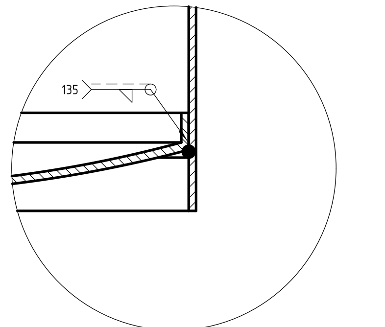
DETALLE D (1:1) Fondo encastrado y pollera fondo a presión con pestaña de 10 contra la pared; filete por debajo
