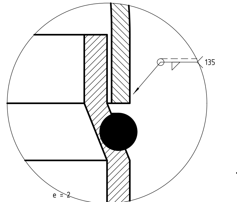
DETALLE C (5:1) Bordón del cuerpo y cúpula escalón e 2 × 5, labio 6 (bordoneadora); cúpula por fuera
