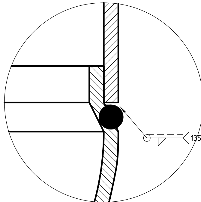
DETALLE D (2:1)
