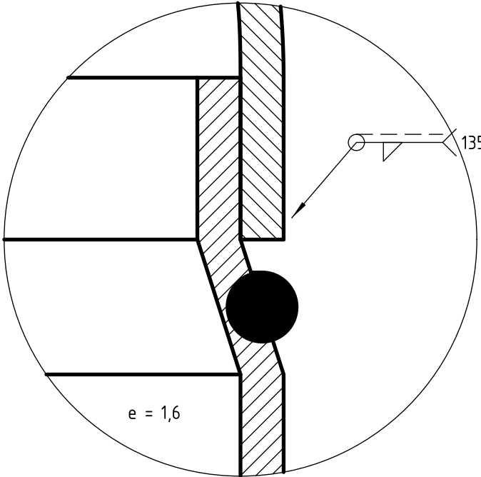
DETALLE C (5:1) Bordón del cuerpo y cúpula escalón e 1,6 × 5, labio 6 (bordoneadora); cúpula por fuera
