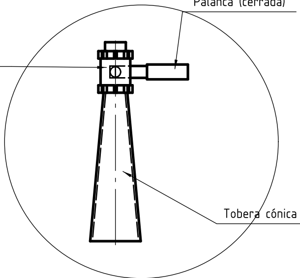
DETALLE E (1:5) Válvula esférica con palanca y tobera
