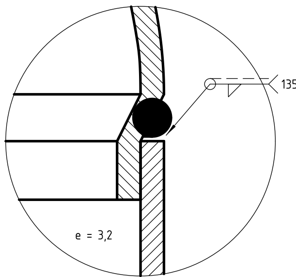
DETALLE C (2:1) Casquete con borde reducido y tope
