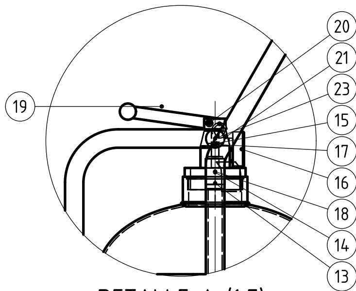
DETALLE A (1:5) Válvula, manómetro y palanca (vista lateral)
