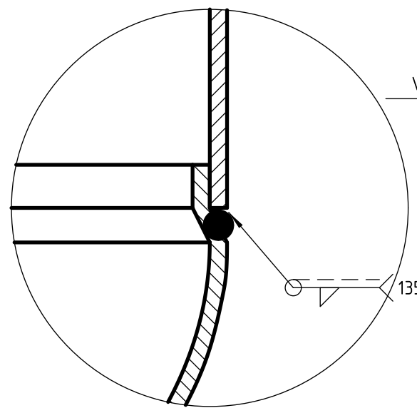
DETALLE D (1:1) Casquete inferior con borde reducido
