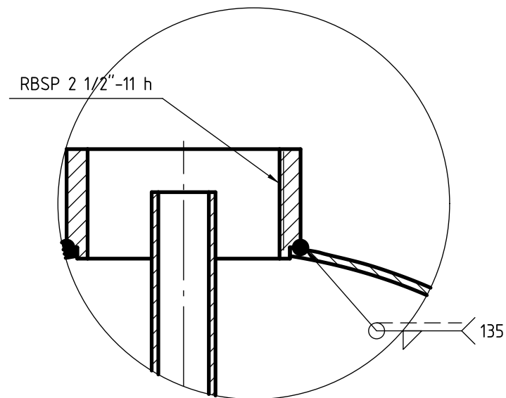
DETALLE B (1:2) Cupla soldada
