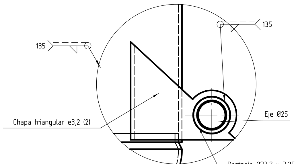
DETALLE F (1:2) Portaeje y chapa triangular (vista lateral, sin rueda)
