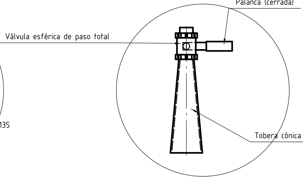
DETALLE E (1:5) Válvula esférica con palanca y tobera
