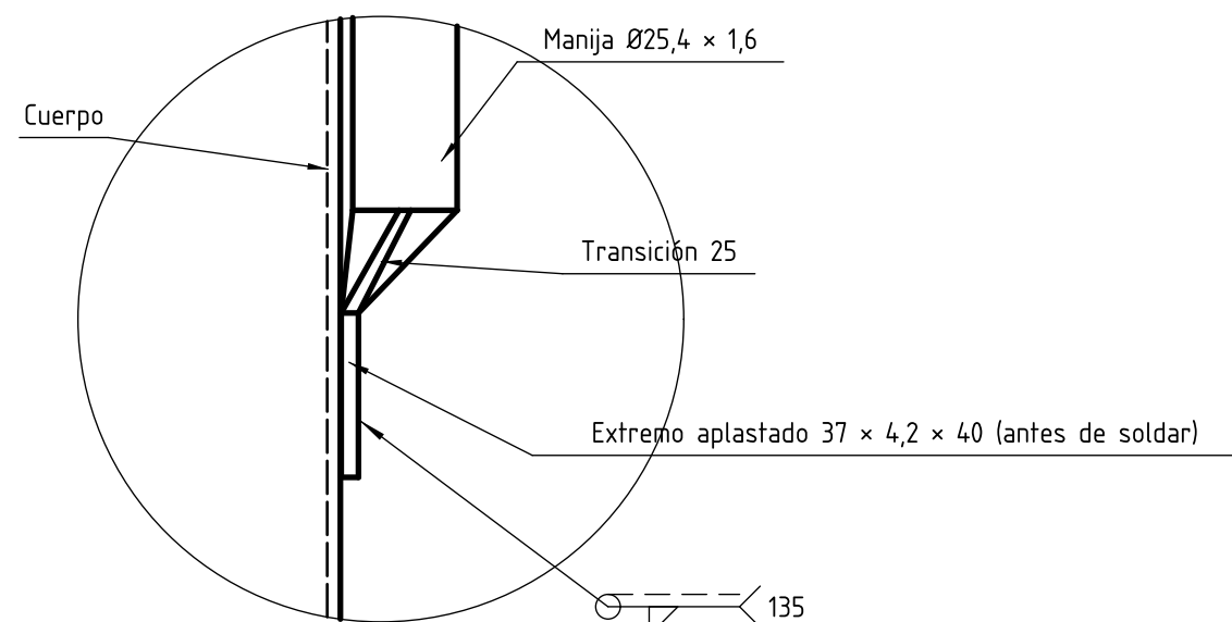
DETALLE G (1:2) Extremo de la pata aplastado y soldado al cuerpo
