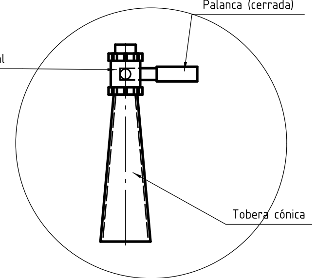
DETALLE E (1:5) Válvula esférica con palanca y tobera
