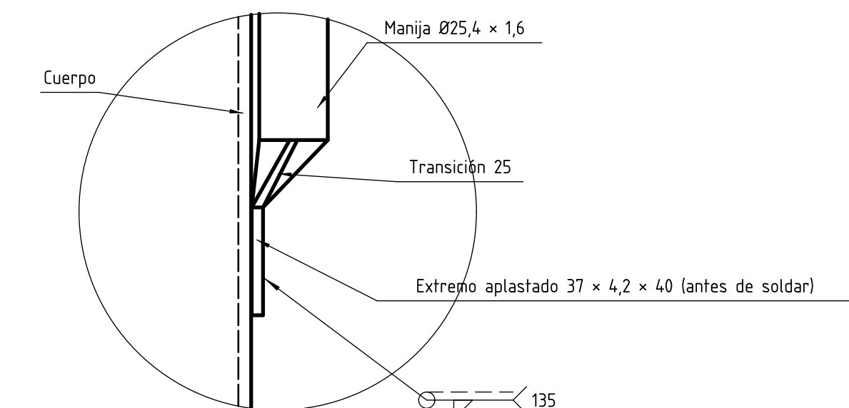
DETALLE G (1:2) Extremo de la pata aplastado y soldado al cuerpo
