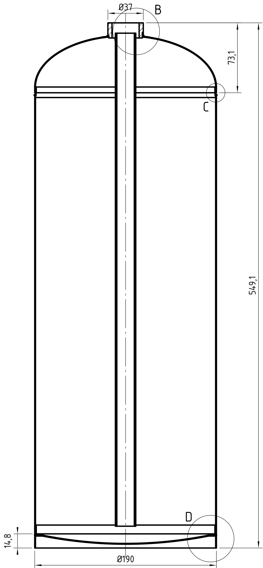
CORTE A-A (1:2)
