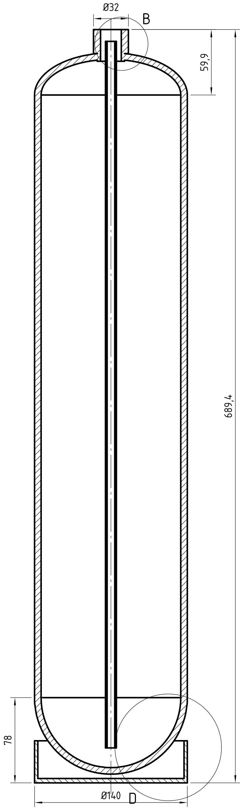
CORTE A-A (1:2)
