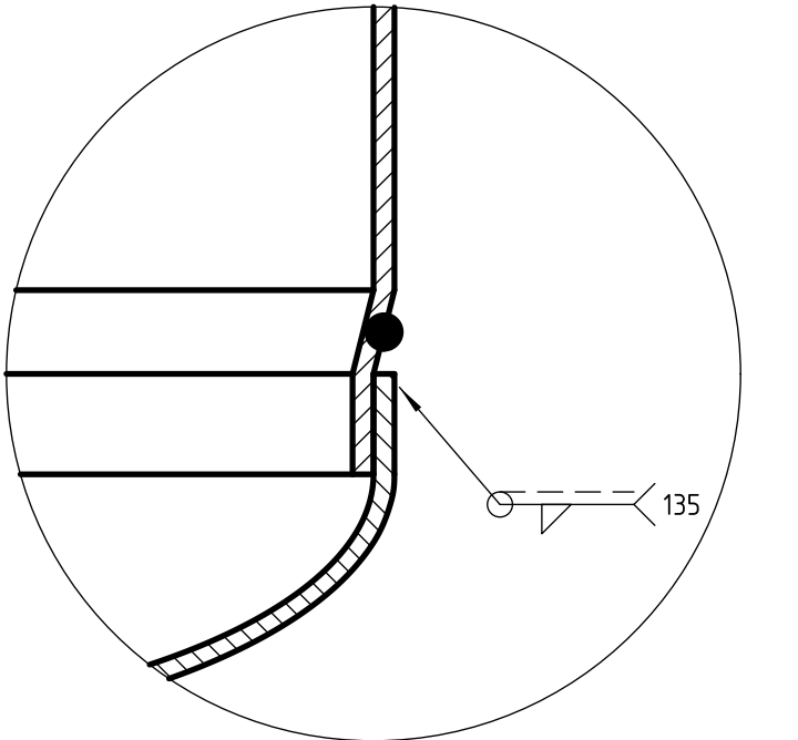
DETALLE D (2:1) Bordón inferior y fondo caño con los dos extremos reducidos: escalón e 1,25 × 5, labio 6
