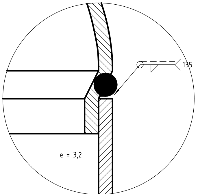
DETALLE C (2:1) Casquete con borde reducido y tope labio 8 dentro del cuerpo, escalón 6,4 × e 3,2; cordón en el escalón
