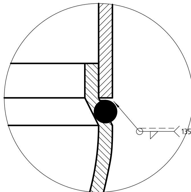
DETALLE D (2:1)
