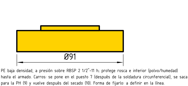
R4 TAPÓN PROTECTOR DE ROSCA
