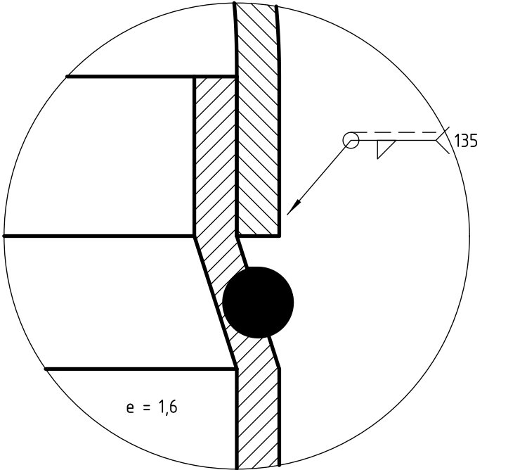
DETALLE C (5:1) Bordón del cuerpo y cúpula escalón e 1,6 × 5, labio 6 (bordoneadora); cúpula por fuera
