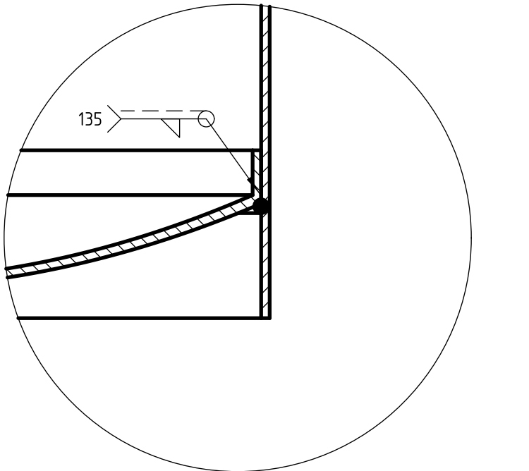
DETALLE D (1:1) Fondo encastrado y pollera fondo a presión con pestaña de 10 contra la pared; filete por debajo
