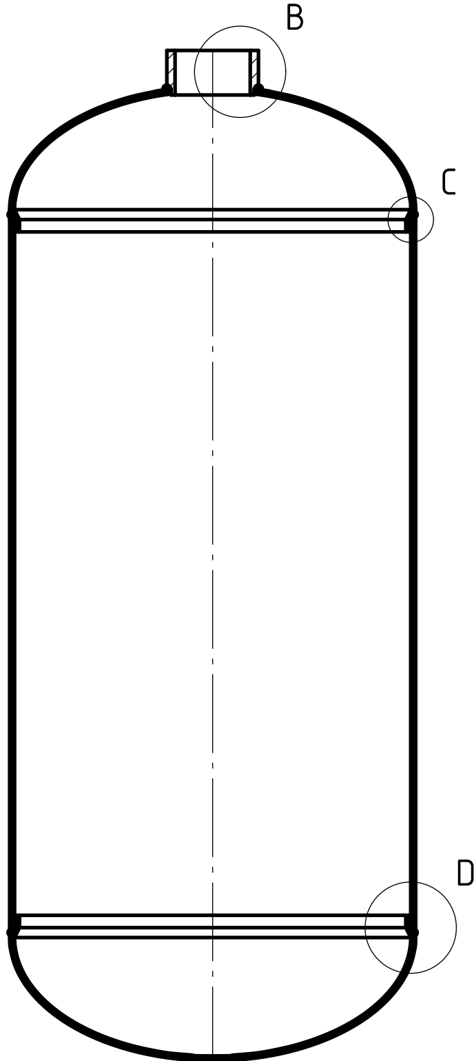
CORTE A-A
