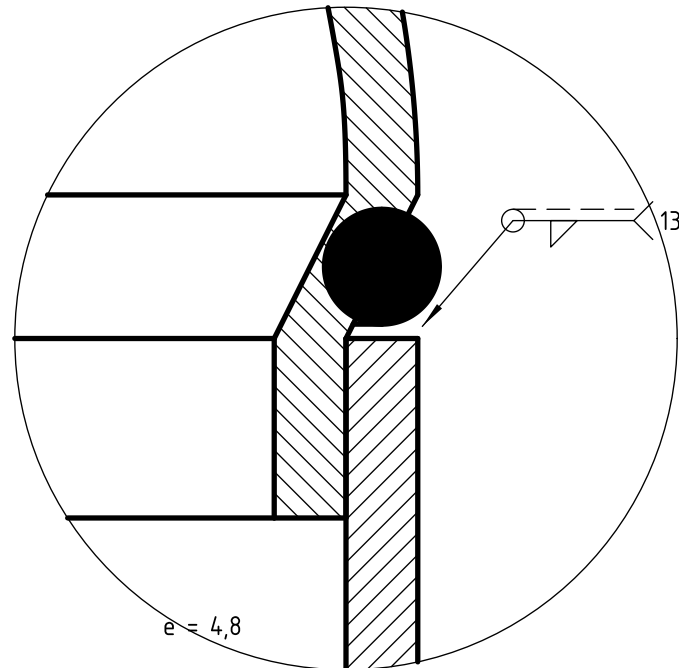
DETALLE C (2:1) Casquete con borde reducido y tope labio 11,9 dentro del cuerpo, escalón 9,5 × e 4,75; cordón en el escalón
