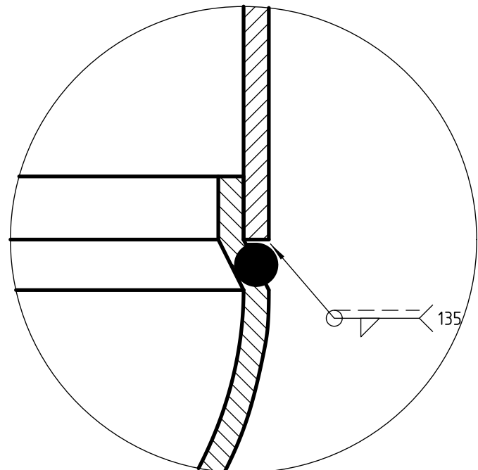
DETALLE D (1:1) Casquete inferior con borde reducido labio 11,9, escalón 9,5; mismo casquete que la cúpula
