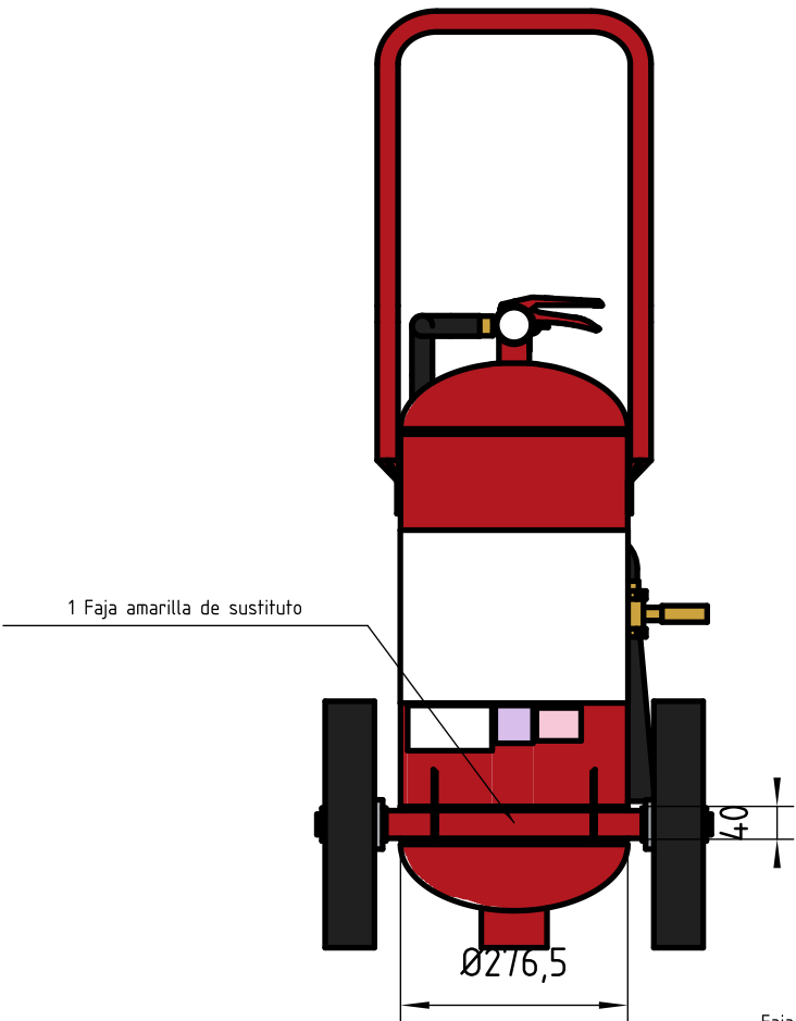
VISTA ANTERIOR (esc. 1:10)
