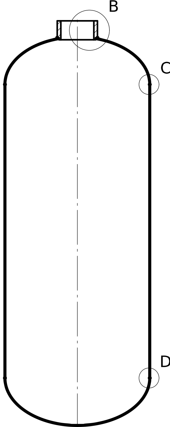
CORTE A-A
