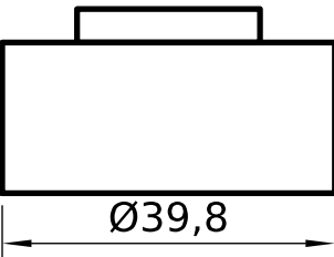
R4 TAPÓN PROTECTOR DE ROSCA
