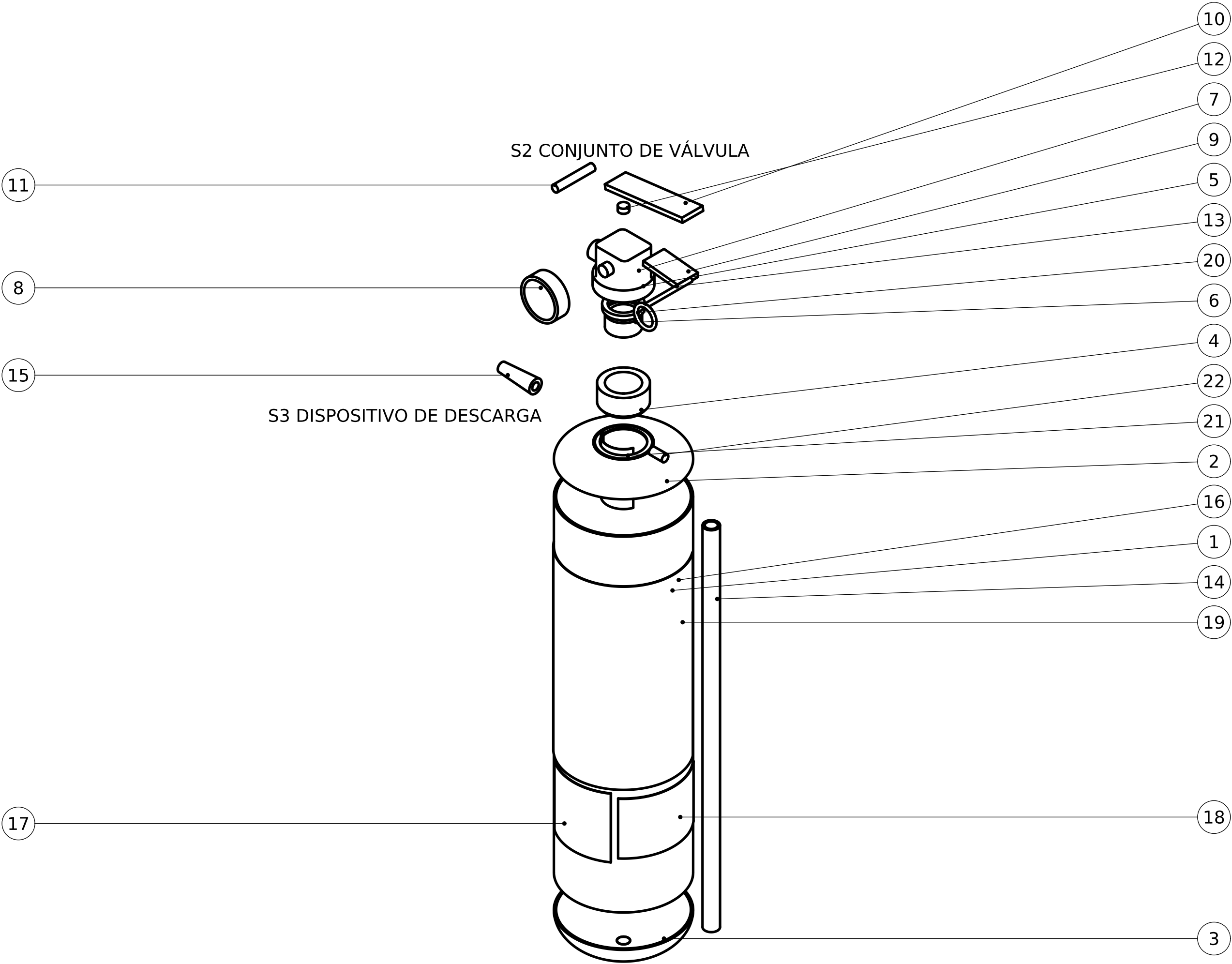
S1 RECIPIENTE (CILINDRO) (FL_REC_ABC_1kg)
