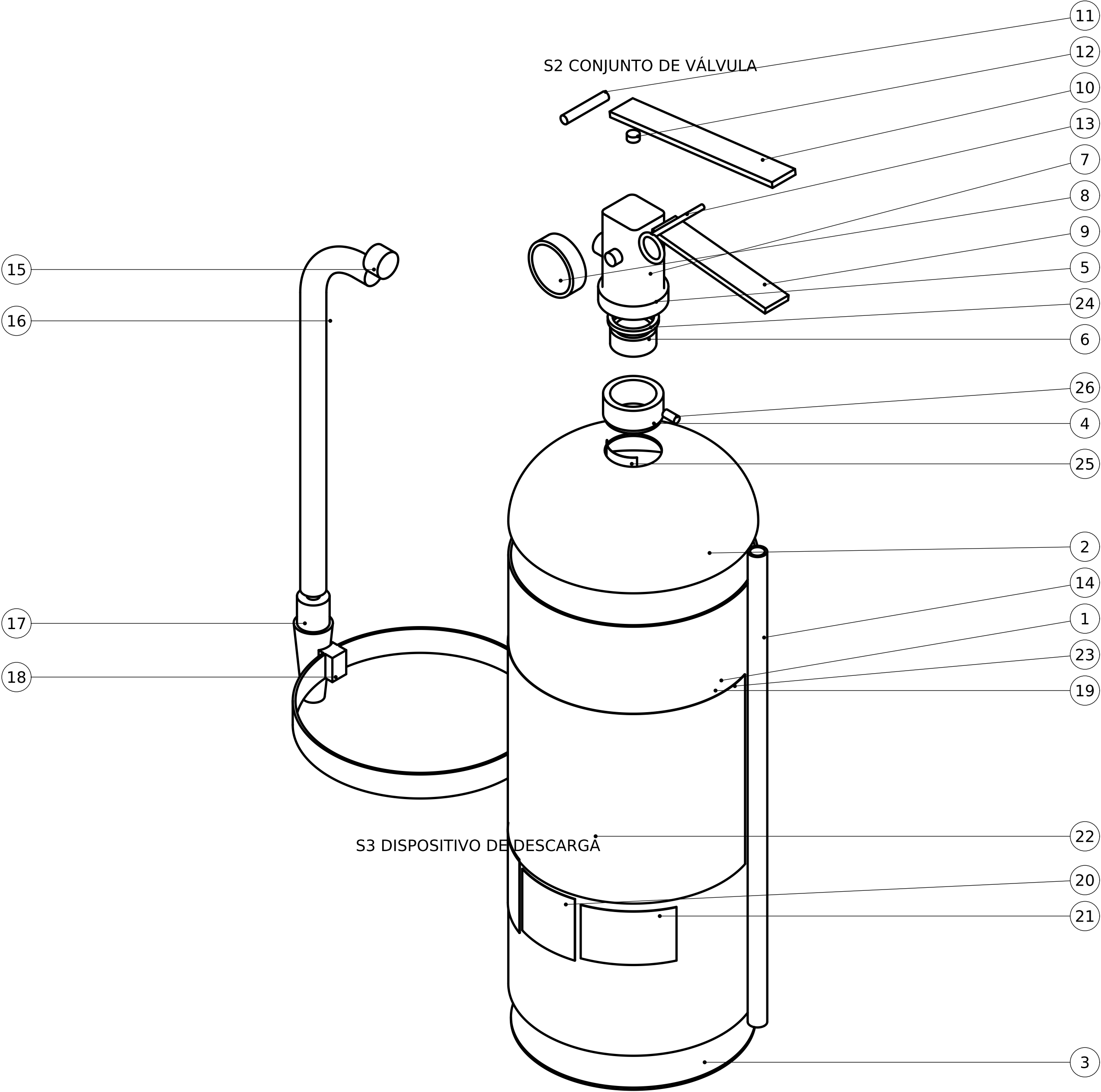
S1 RECIPIENTE (CILINDRO) (FL_REC_ABC_5kg)
