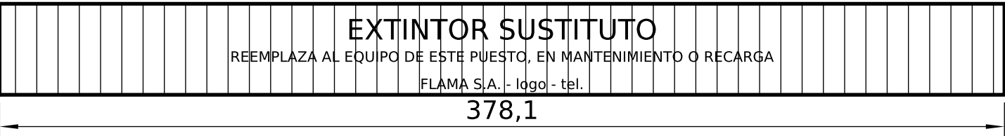
DETALLE 1 - DESARROLLO DE LA FAJA 34 × 378 (esc. 1:2) - amarillo; leyendas negras repetidas
