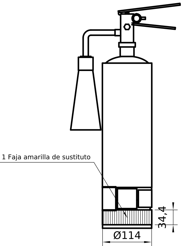
VISTA ANTERIOR (esc. 1:5)
