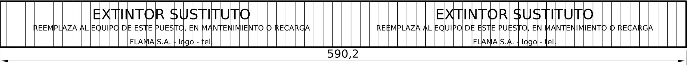
DETALLE 1 - DESARROLLO DE LA FAJA 40 × 590 (esc. 1:2) - amarillo; leyendas negras repetidas
