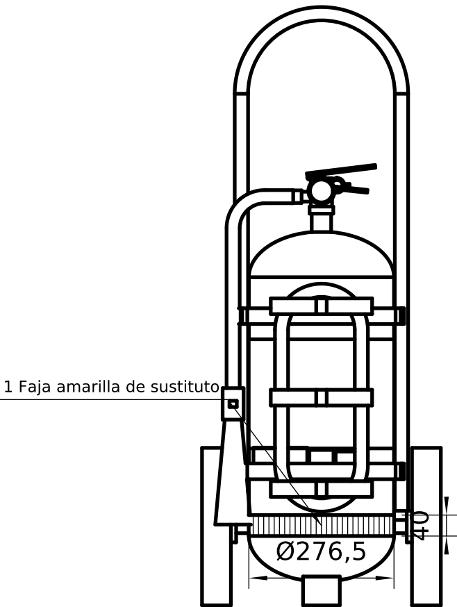
VISTA ANTERIOR (esc. 1:10)
