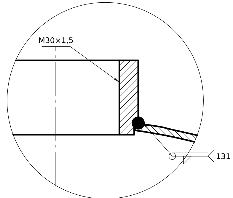
DETALLE B (2:1) Cuello roscado
