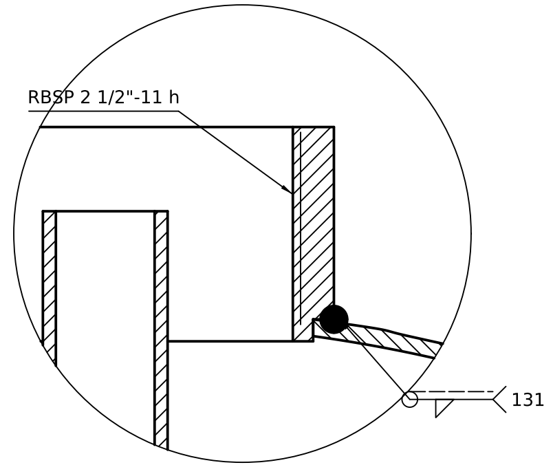
B (1:1) Cuello roscado
