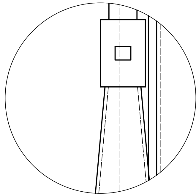
E (1:2) Válvula esférica y tobera
