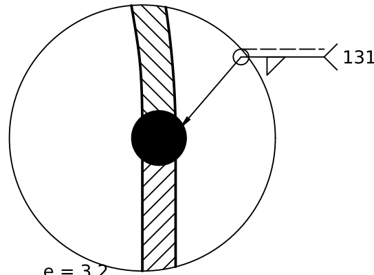
C (2:1) Unión cúpula-cuerpo
