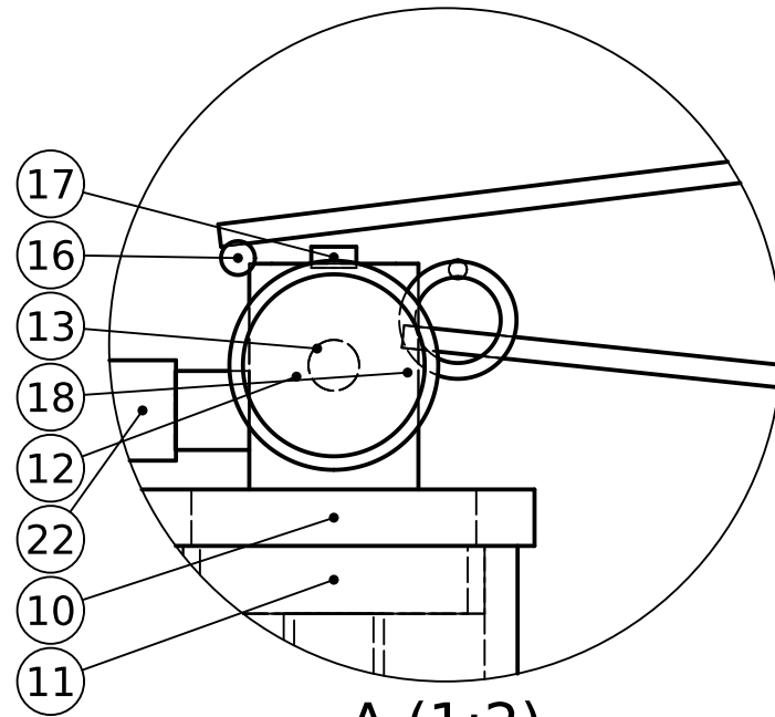
A (1:2) Válvula, manómetro y manijas
