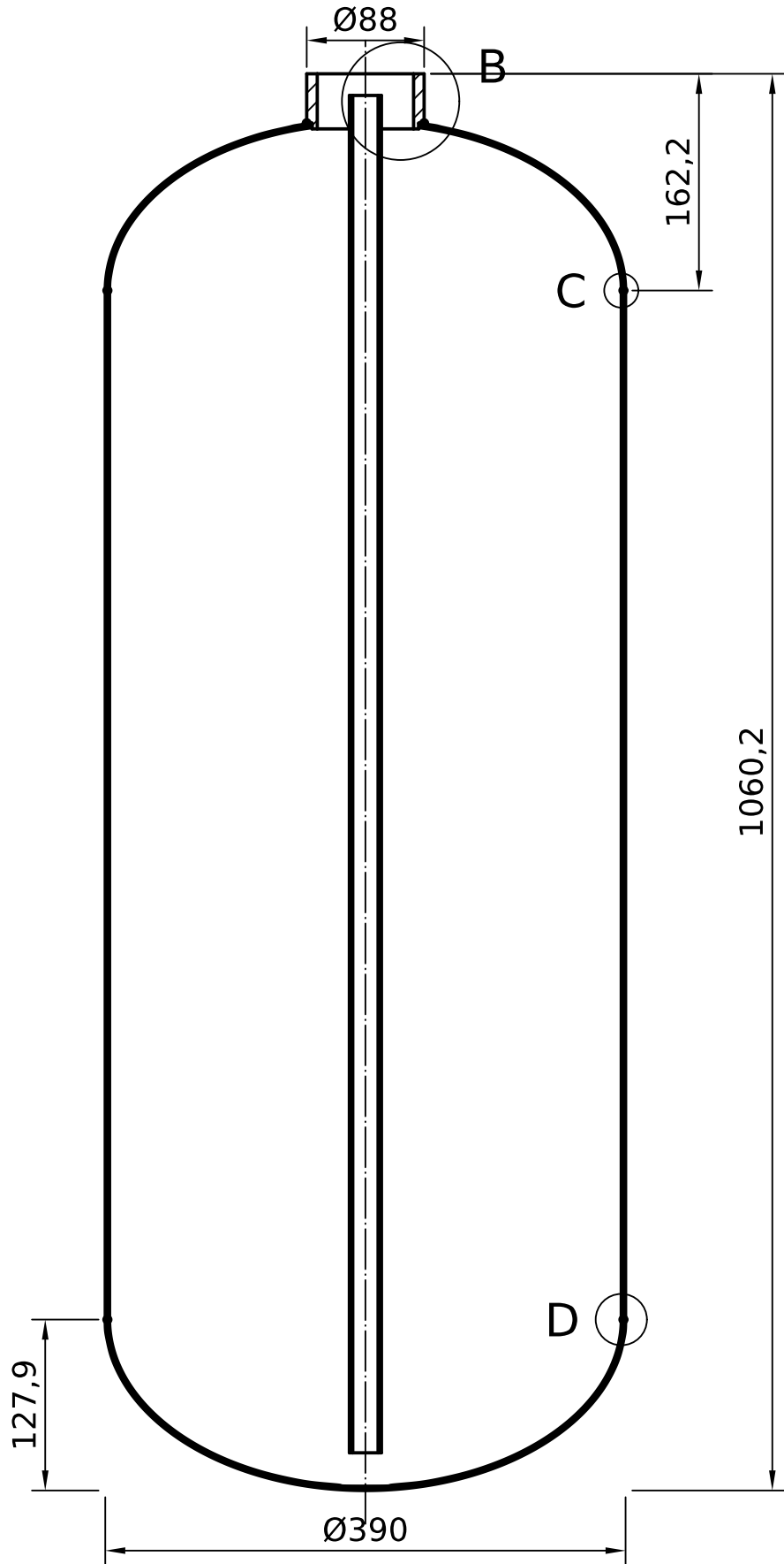
A-A (1:5)
