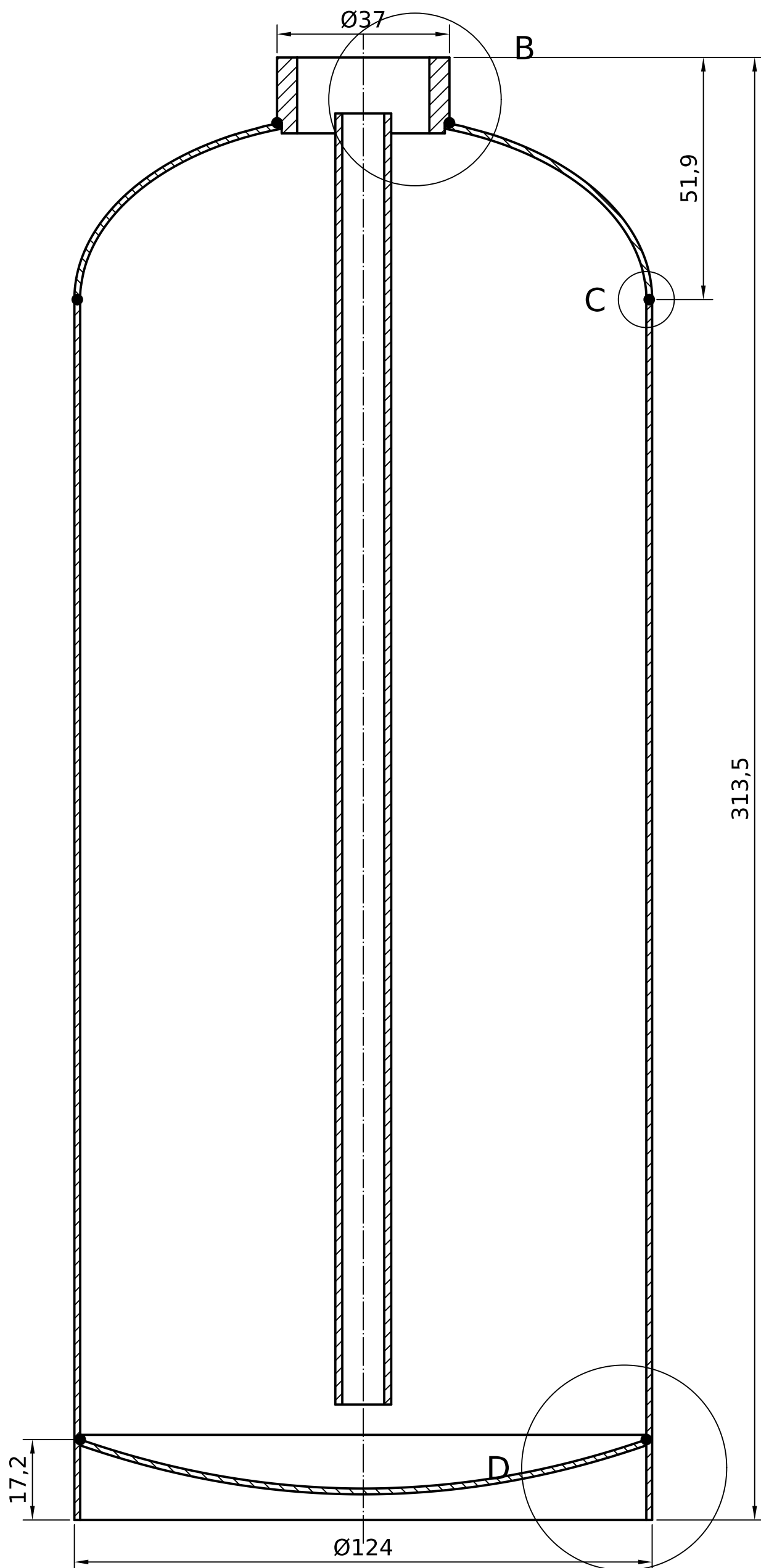
A-A (1:1)
