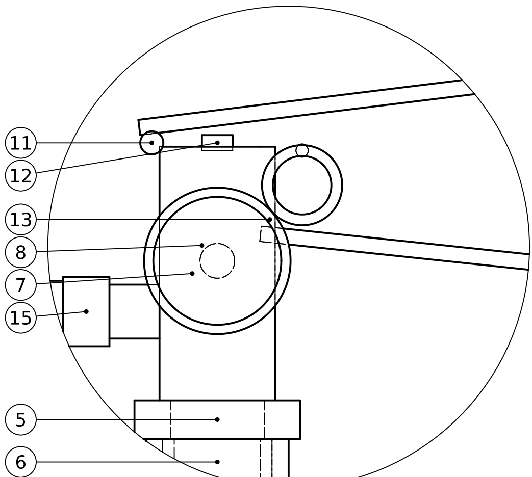
A (1:1) Válvula, manómetro y manijas
