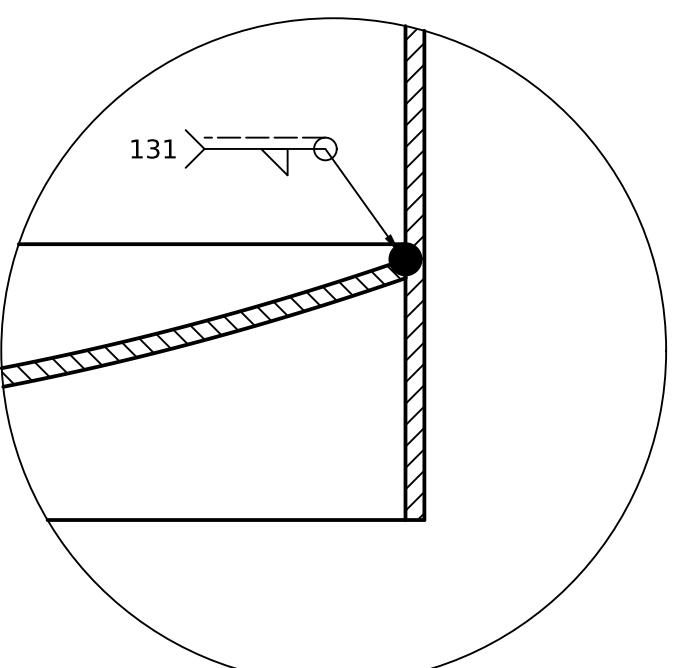
D (2:1) Fondo y pollera
