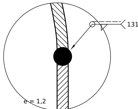
C (5:1) Unión cúpula-cuerpo
