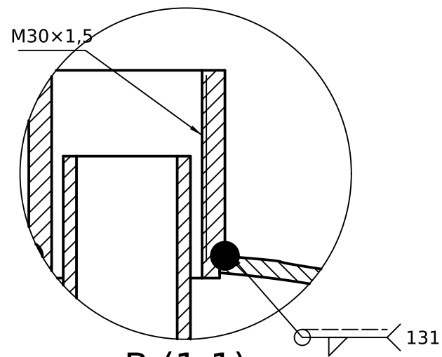
B (1:1) Cuello roscado
