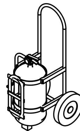
ISOMETRÍA (1:20)
