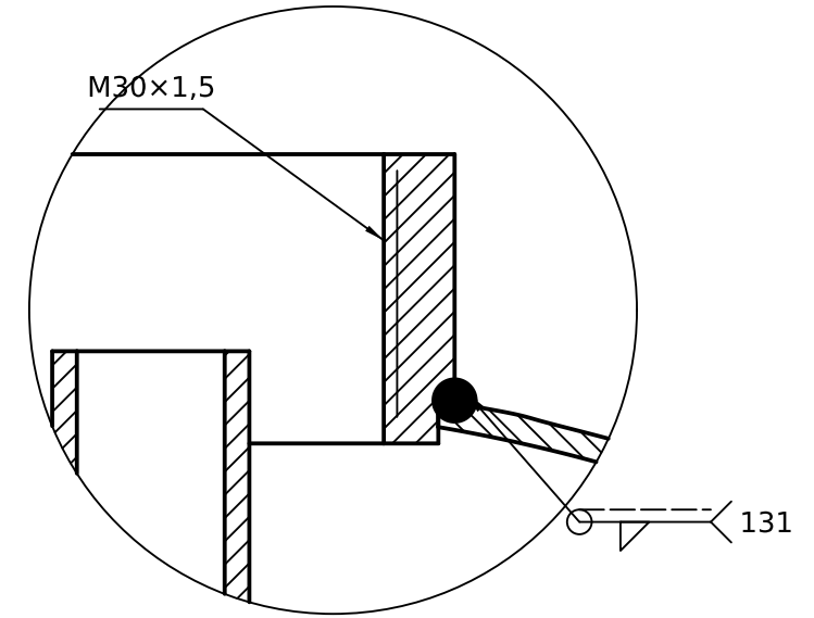
B (2:1) Cuello roscado
