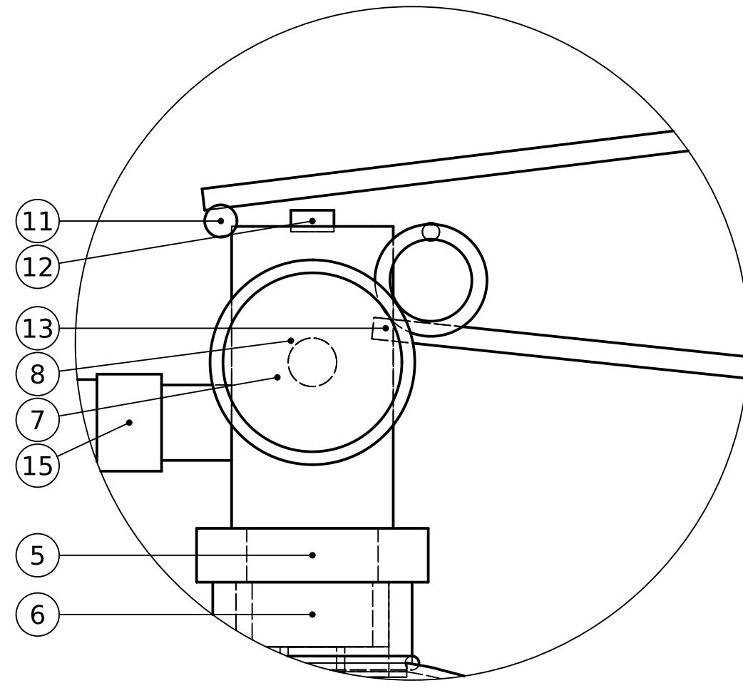
A (1:1) Válvula, manómetro y manijas
