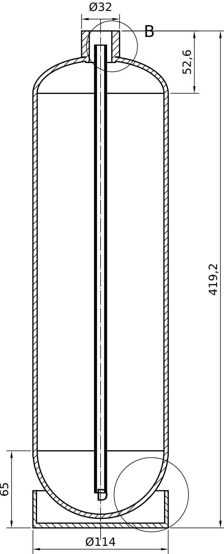
A-A (1:2)
