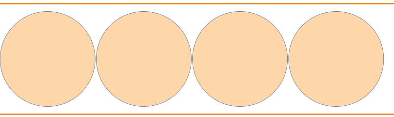
Cúpula 10 kg: Ø 258 en fleje 2,00 × 300 - paso 261,0 - aprovech. 66,8 %
