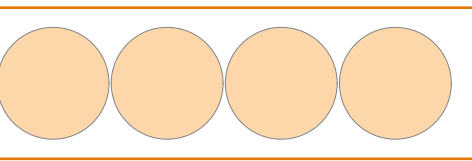
Fondo 2,5 kg: Ø 148 en fleje 1,25 × 200 - paso 151,0 - aprovech. 57,0 %
