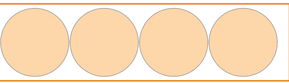
Fondo 5 kg: Ø 177 en fleje 1,60 × 200 - paso 180,0 - aprovech. 68,3 %
