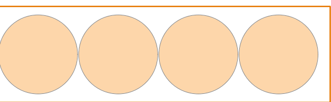
Fondo 10 kg: Ø 205 en fleje 2,00 × 249 - paso 208,0 - aprovech. 63,7 %
