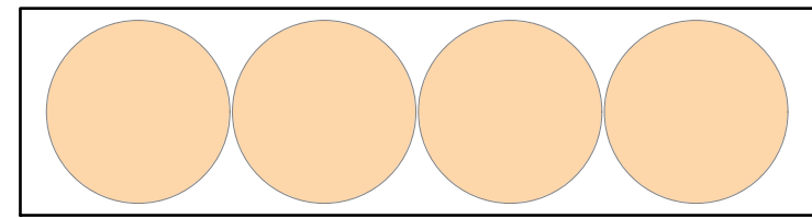
Cúpula 5 kg: Ø 221 en fleje 1,60 × 250 - paso 224,0 - aprovech. 68,5 %
