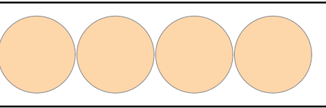
Fondo 2,5 kg: Ø 148 en fleje 1,25 × 200 - paso 151,0 - aprovech. 57,0 %
