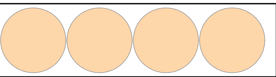
Fondo 5 kg: Ø 177 en fleje 1,60 × 200 - paso 180,0 - aprovech. 68,3 %
