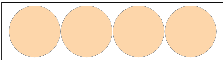
Cúpula 5 kg: Ø 221 en fleje 1,60 × 250 - paso 224,0 - aprovech. 68,5 %
