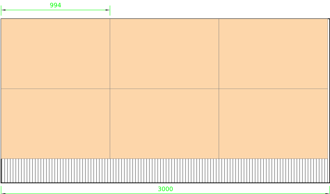
Cuerpo 50 kg - hoja LAC 3,20 × 1500 × 3000
