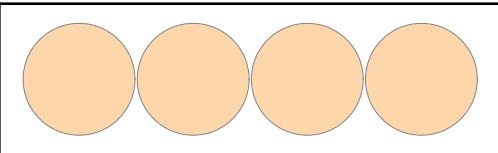
Fondo 2,5 kg: Ø 148 en fleje 1,25 × 200 - paso 151,0 - aprovech. 57,0 %
