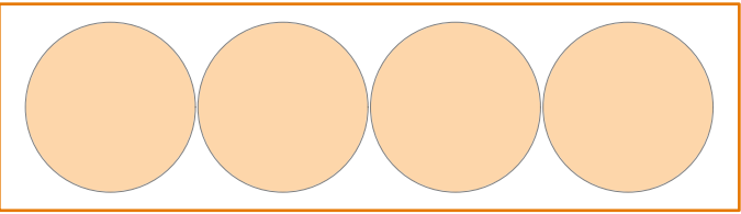
Fondo 10 kg: Ø 205 en fleje 2,00 × 249 - paso 208,0 - aprovech. 63,7 %
