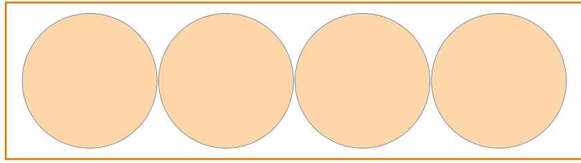
Cúpula 10 kg: Ø 258 en fleje 2,00 × 300 - paso 261,0 - aprovech. 66,8 %
