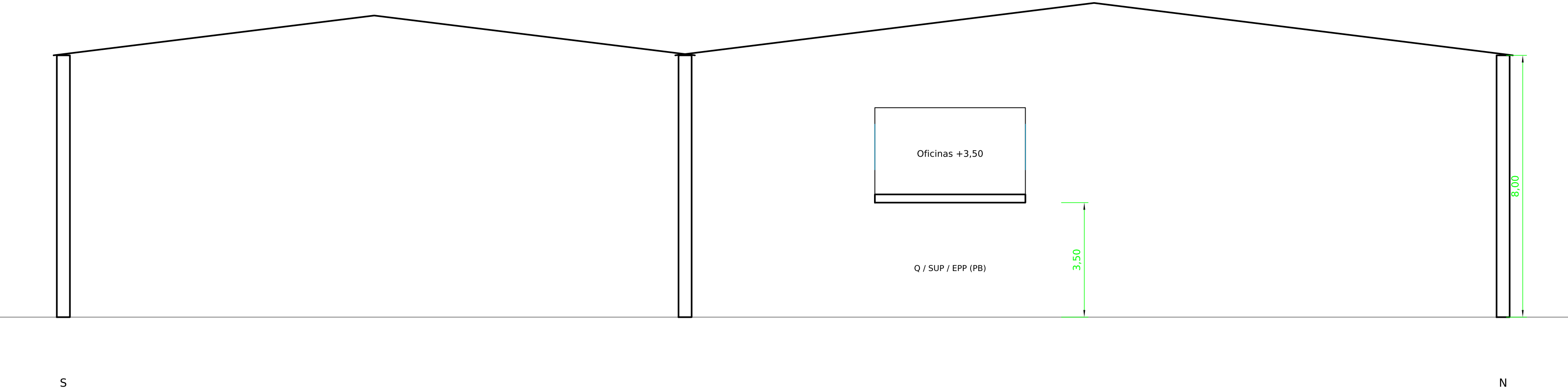
CORTE B-B POR EL ENTREPISO (x = 55 m) - 1:100
