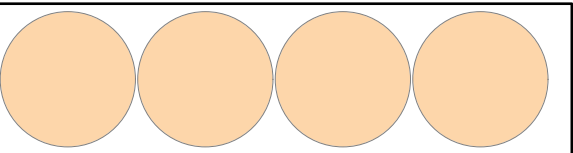
Cúpula 2,5 kg: Ø 179 en fleje 1,25 × 200 - paso 182,0 - aprovech. 69,1 %
