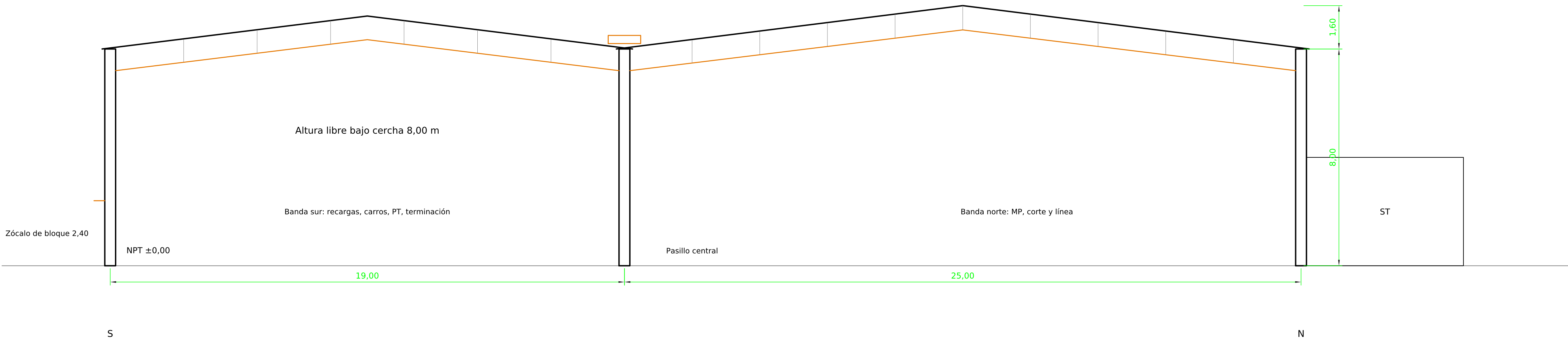
CORTE TRANSVERSAL A-A (por eje 4) - 1:100
