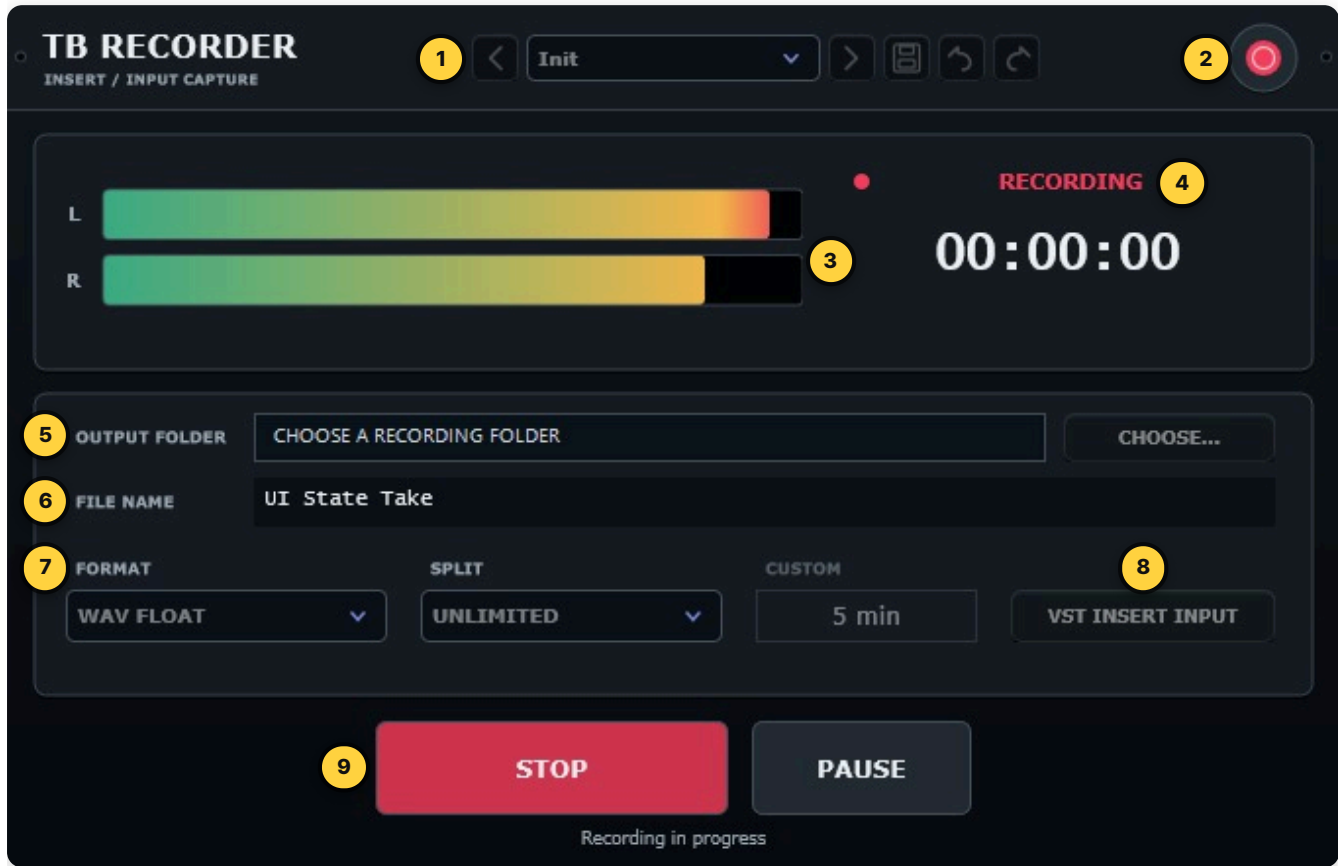
녹음 중인 TB Recorder 1.0 화면.
