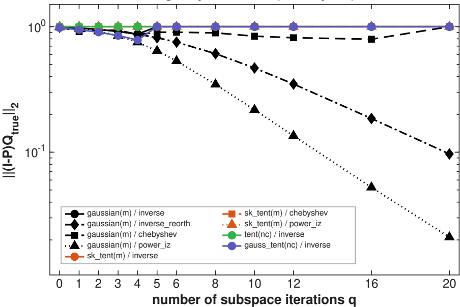
eigenspace error ( Z = T_{\text{sym}}^{-1} )
