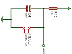
RESET DEVRESİ
