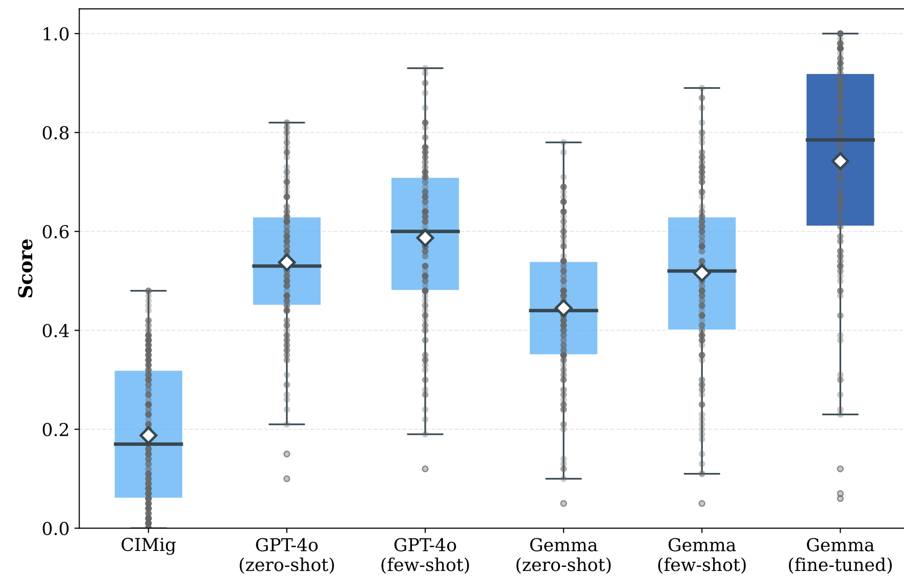
CrystalBLEU
