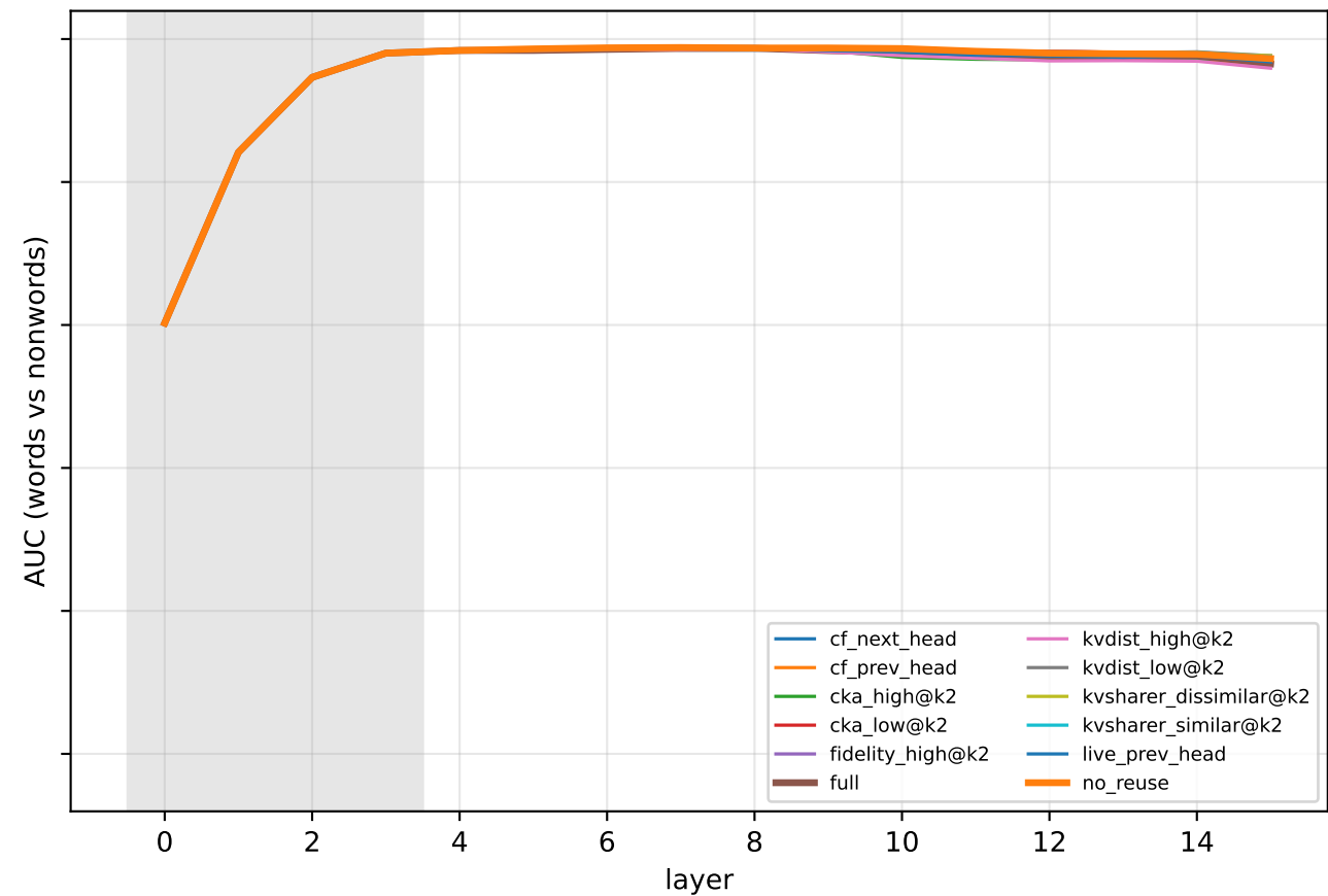
Llama-3.2-1B: retrained readout
