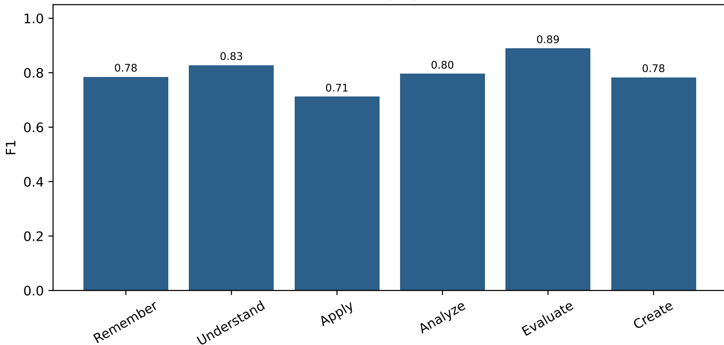
Per-class F1 (deployable model)
