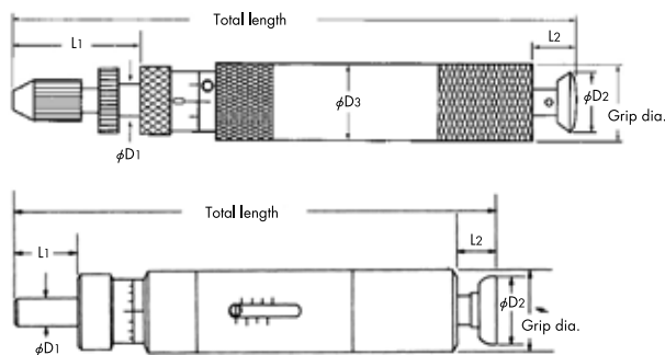
CN15,CN30LTDK(N·m Unit)
