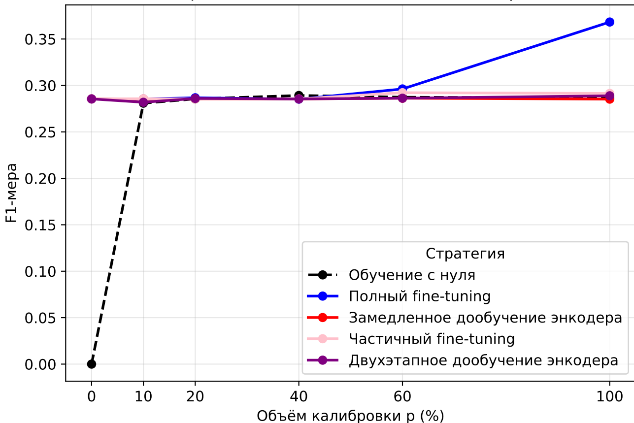
F1-мера в зависимости от объёма калибровки
