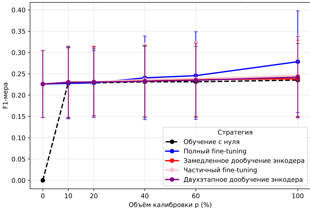
F1-мера в зависимости от объема калибровки
