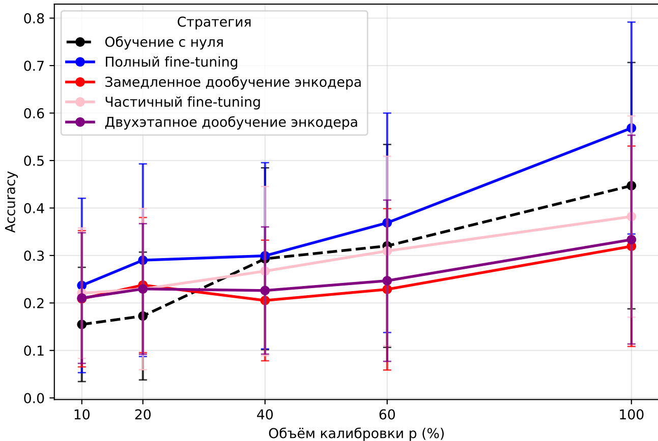
Ассурасу в зависимости от объёма калибровки
