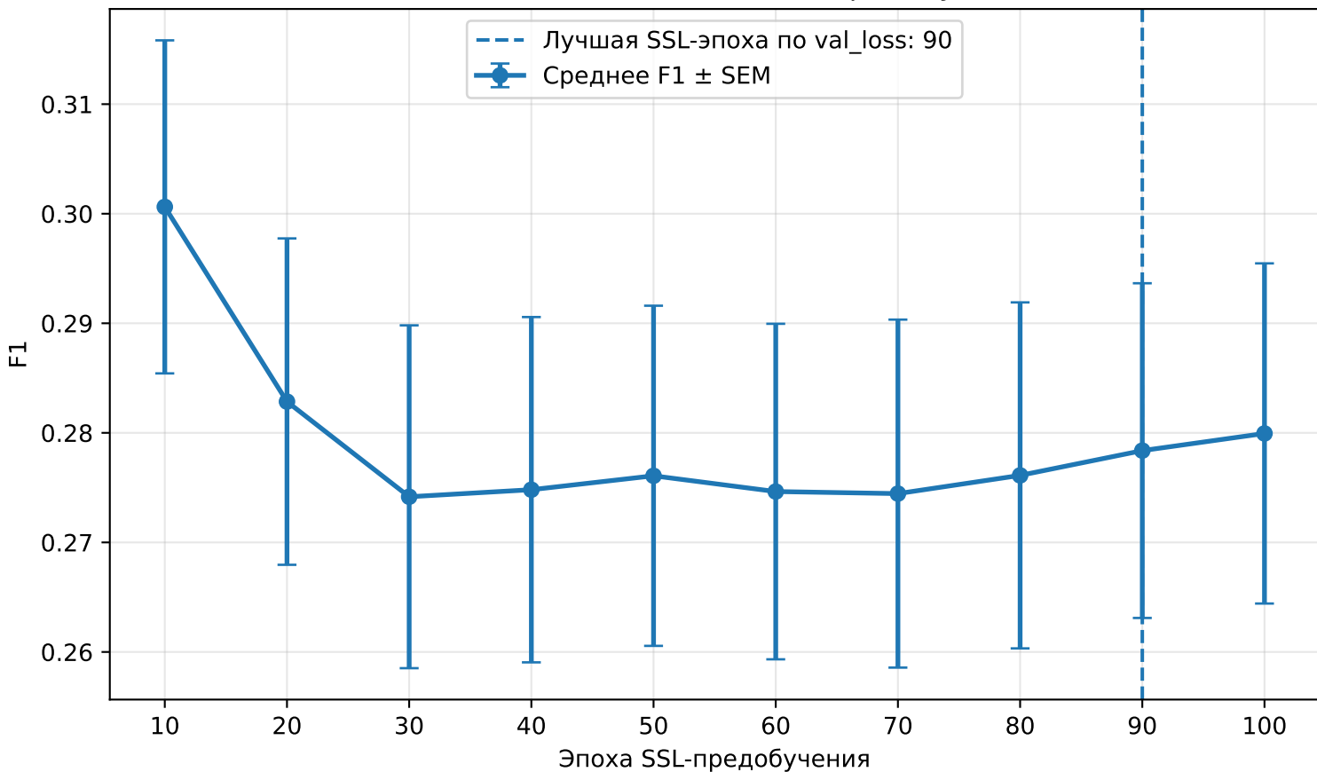
Зависимость F1 от эпохи SSL-предобучения
