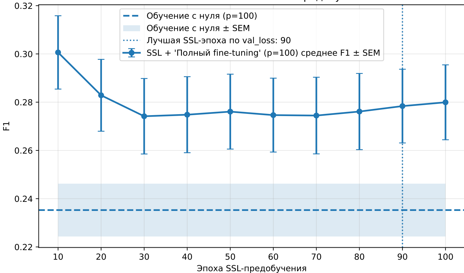
F1 в зависимости от эпохи SSL-предобучения
