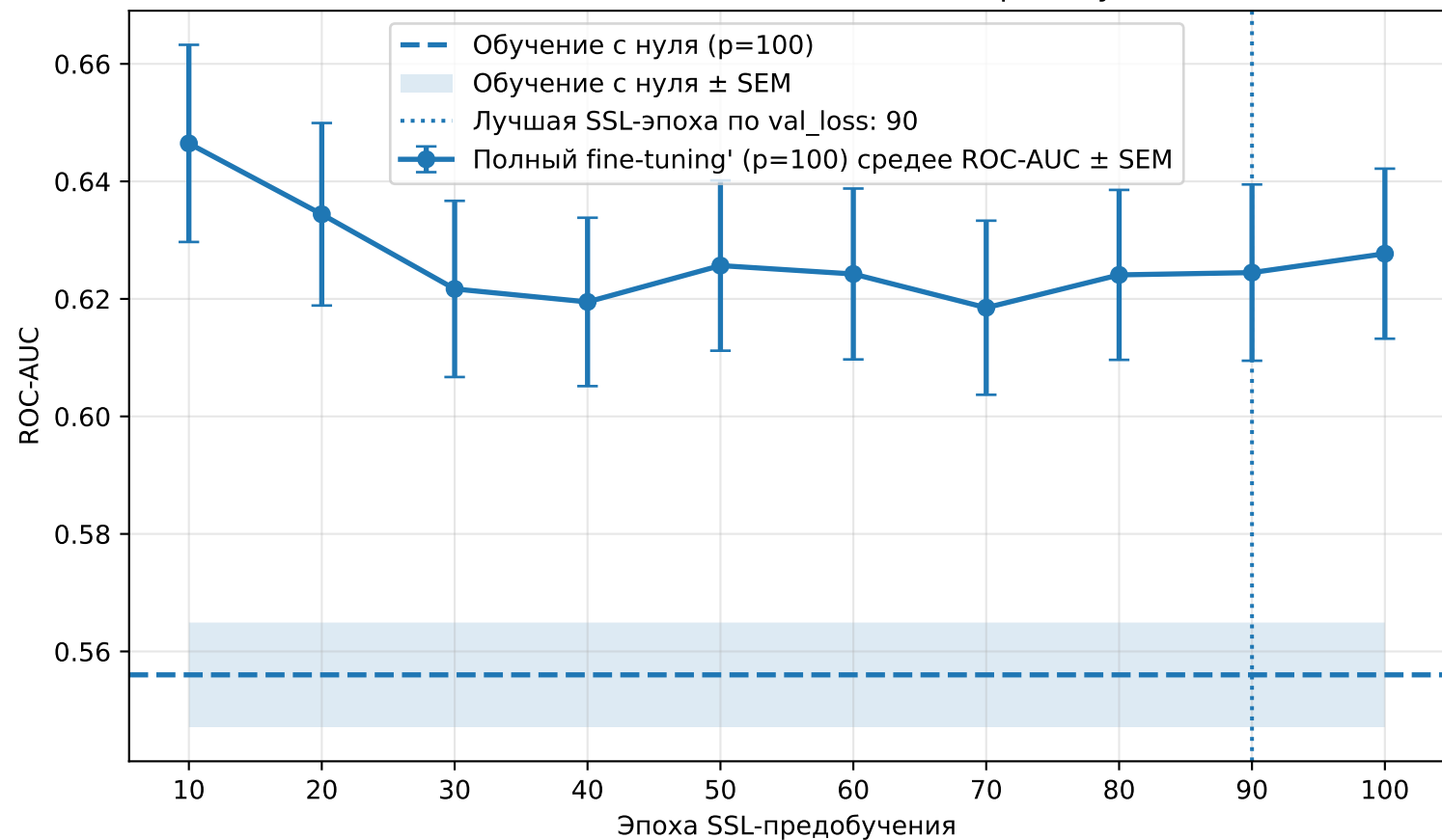
ROC-AUC в зависимости от эпохи SSL-предобучения
