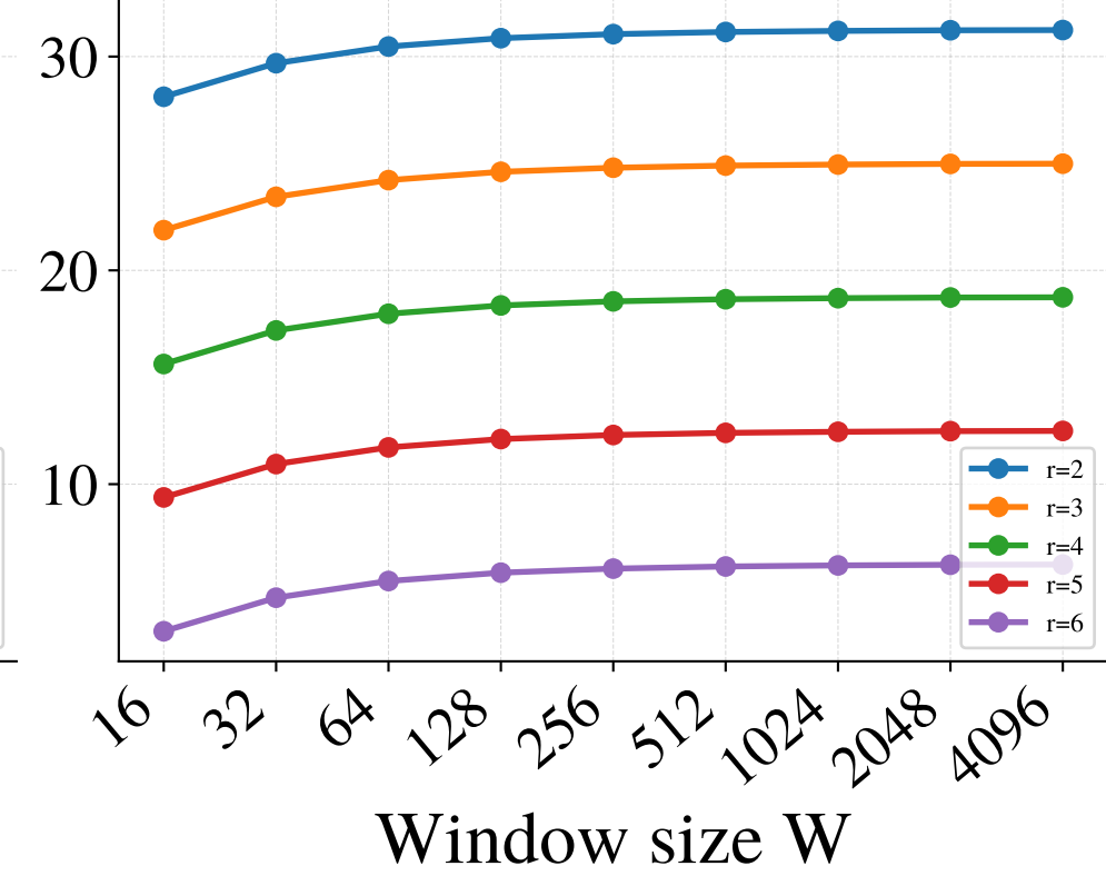
TinyLlama-1.1B
