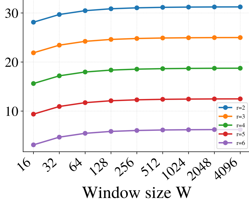
Phi-2
