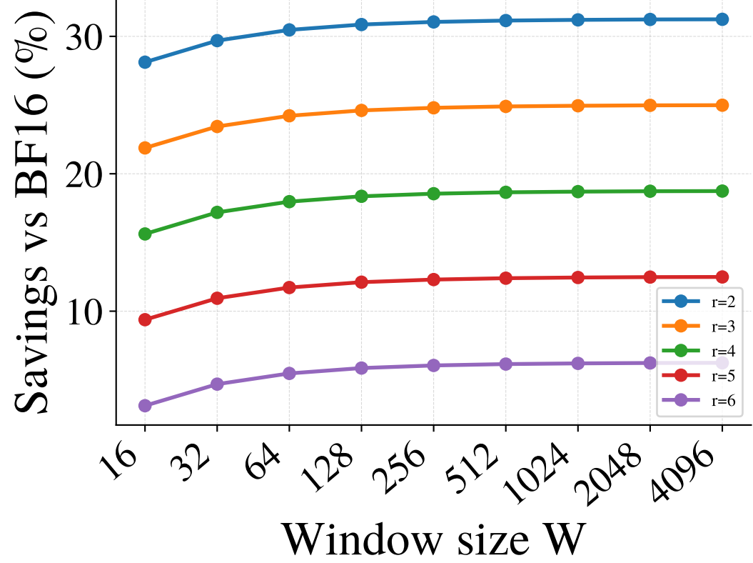
Mistral-7B
